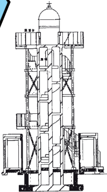
断面図
