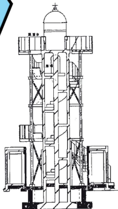
断面図
