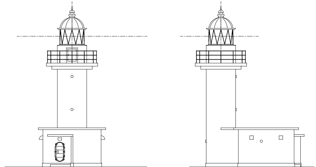
灯台姿図 1/200
