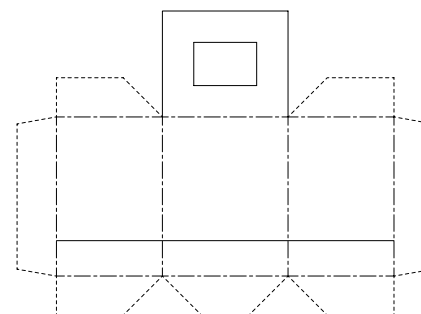
天水溜桝
